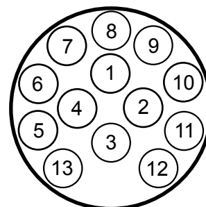
DIN/ISO 11446 13-pol
